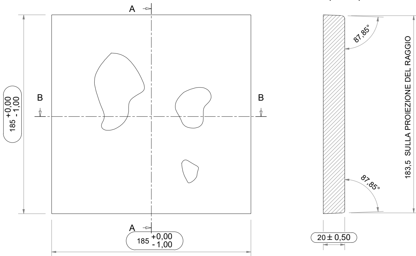
A-A (1 : 2)
